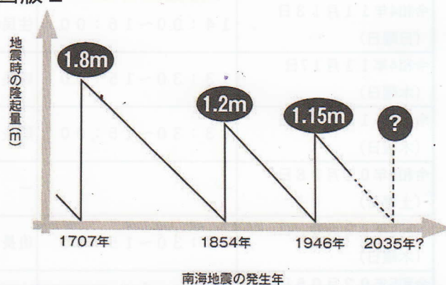
図版2 室津港の地震隆起
