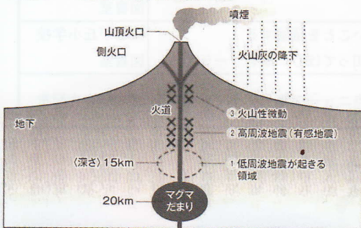
図版3 富士山の地下構造と断面図
