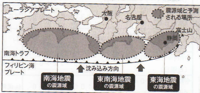
図版1 南海トラフ沿いで周期的に起きる巨大地震
