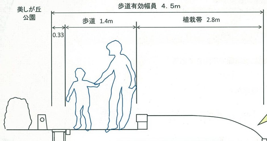
現況図 (A-A断面)
